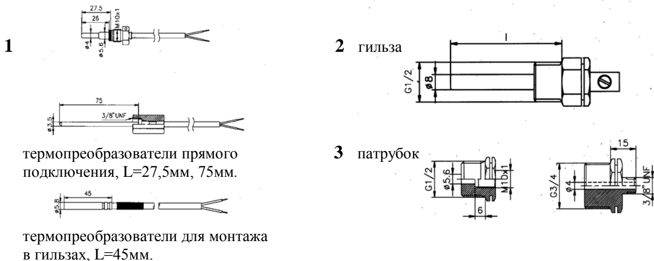
Рис 2. Термопреобразователи сопротивления.
