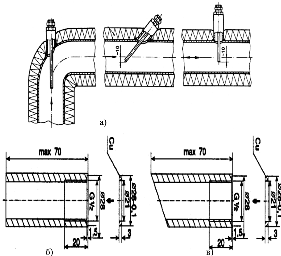
Рис 3. Монтаж термopеобразователей сопротивления.
